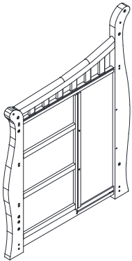
(H) Middle Panel (x1) (H) Panneau du milieu (x1)
